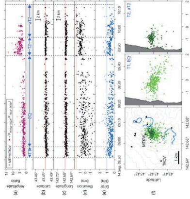
図1. 2020年9月の地盤変動イベントで見られた地震活動域の浅部への移動 (Permana and Aoyama, 2022).
