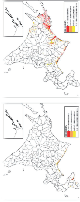
日本海溝モデルによる土砂災害危険ランク 千島海溝モデルによる土砂災害危険ランク
