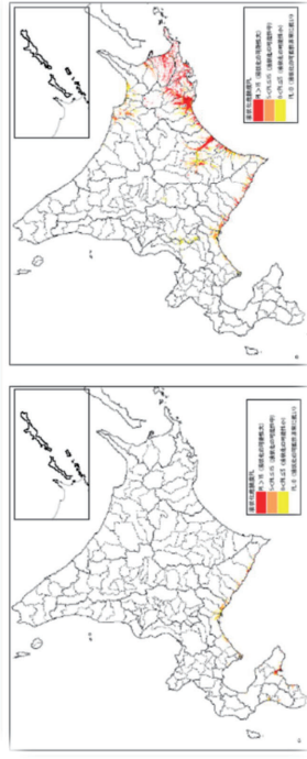
日本海溝モデルによる液状化危険度 千島海溝モデルによる液状化危険度
